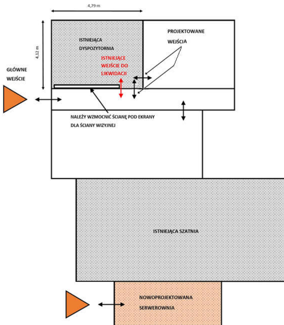
Rys. 1 Szkic przyjętego wariantu rozbudowy istniejącego budynku administracyjno-socjalnego na potrzeby dyspozytorni i serwerowni
