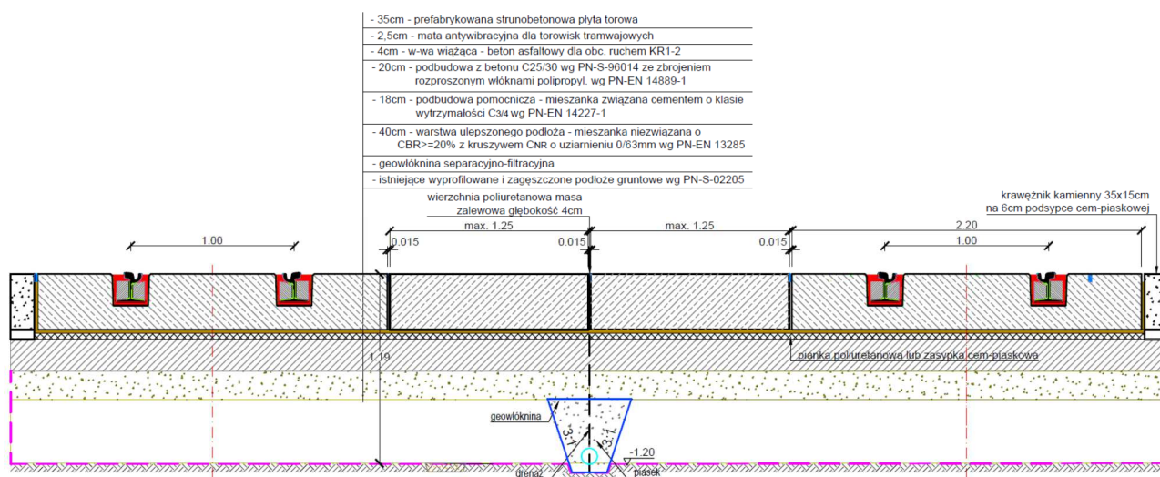
Rysunek 4. – Proponowana / poglądowa konstrukcja torowiska z prefabrykowanych żelbetonowych płyt torowych.
