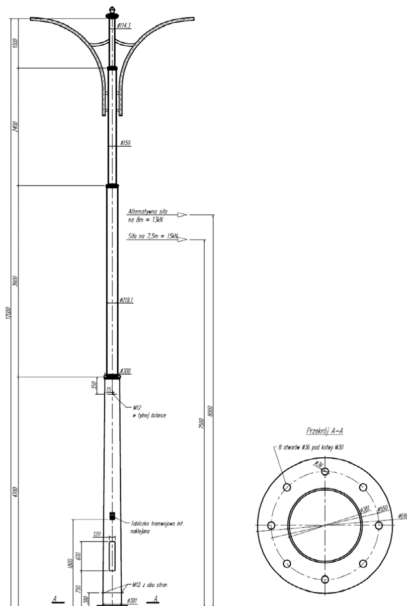
Rysunek 5. Sylwetka słupa stalowego trakcyjno – oświetleniowego o przekroju rurowym na terenie Miasta Pabianice.
