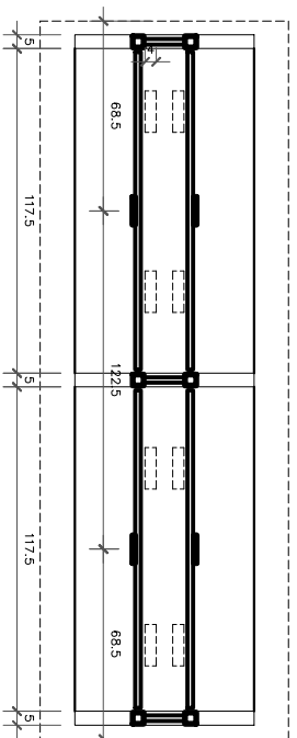
PRZEKRÓJ A-A
